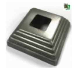
Основание балясины, арт. R10436.02 80x80x1мм, кв.25x25мм Вес: 0.075 кг Цена (за шт): 10 руб.
